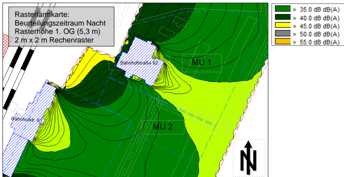
Abbildung 13 Rasterlärnkarte Schienenverkehr 'OHE-Gelände' (Ausschnitt ohne Maßstab)
