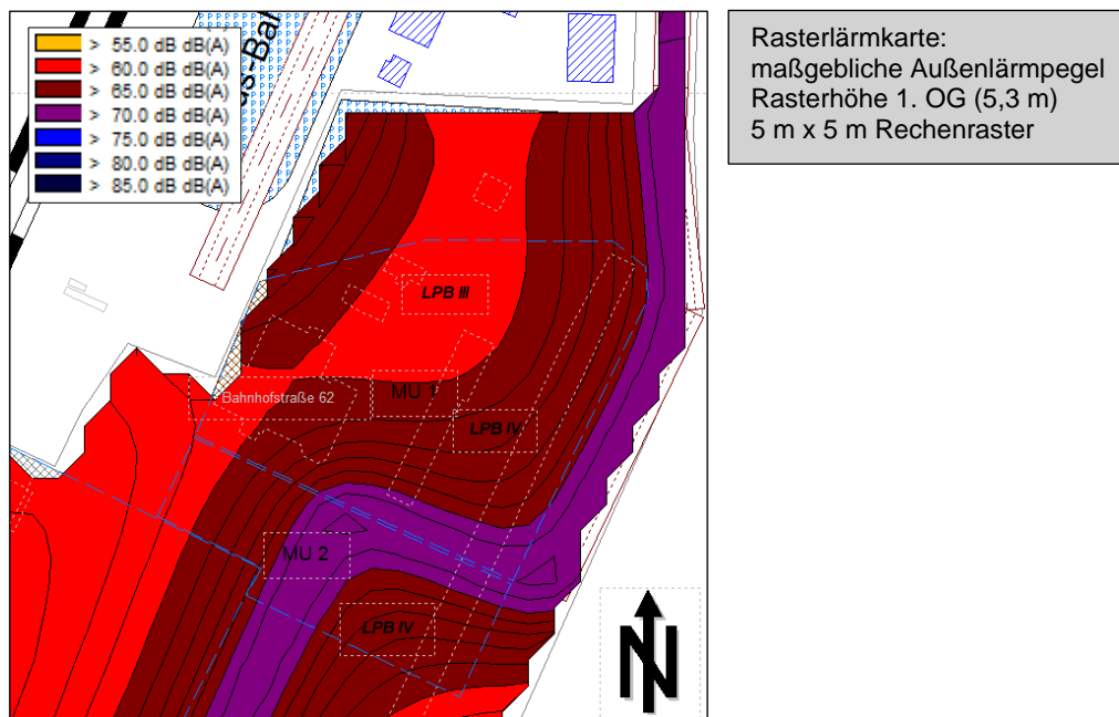
Abbildung 15 Lärmpegelbereiche Plangebiet 'OHE-Gelände' (Ausschnitt ohne Maßstab)
