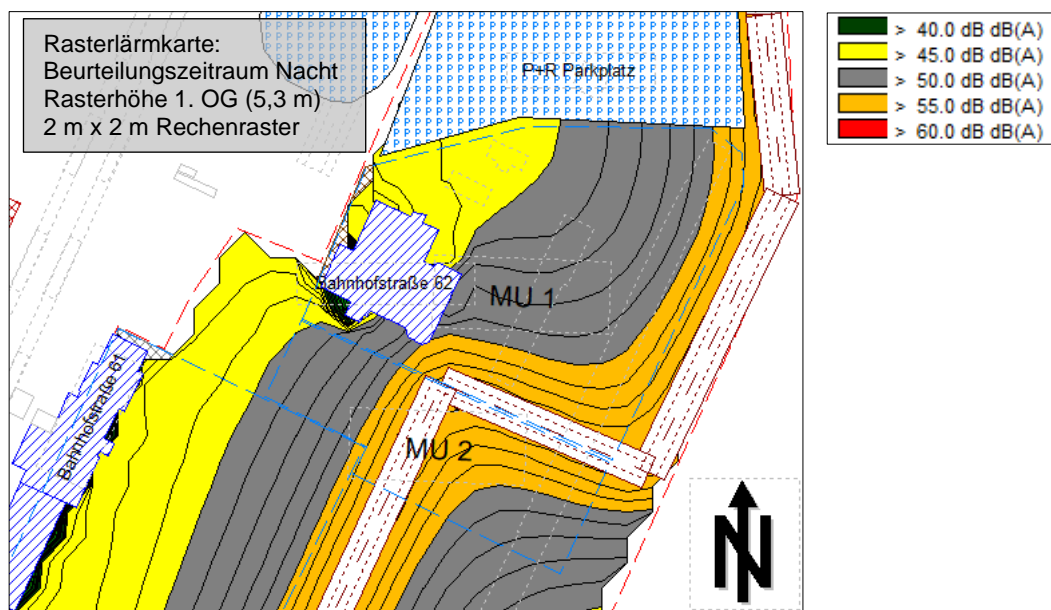
Abbildung 14 Rasterlärnkarte Straßenverkehr 'OHE-Gelände' (Ausschnitt ohne Maßstab)
